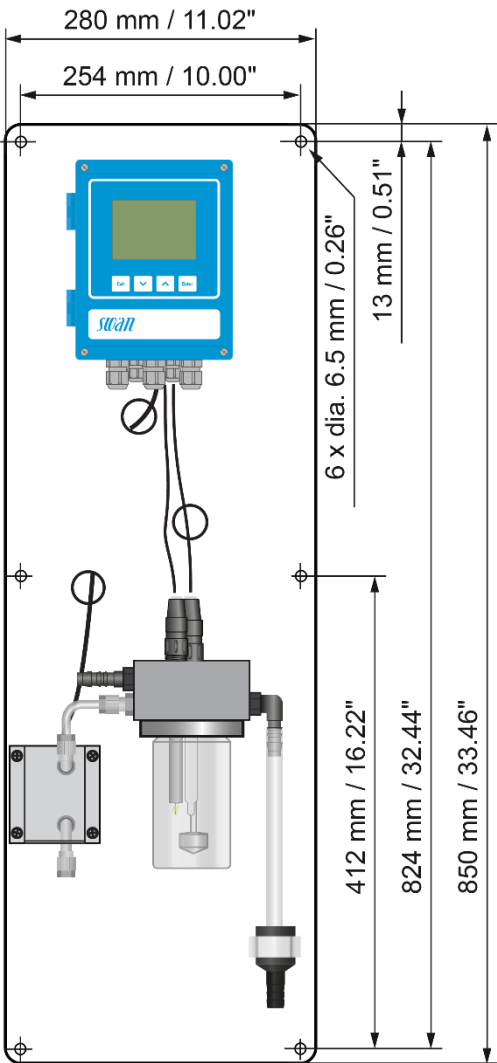
Monitor AMI-II pH/Redox M-Flow con sensor U-Flow Swansensor opcional y boquilla de pulverización opcional.
